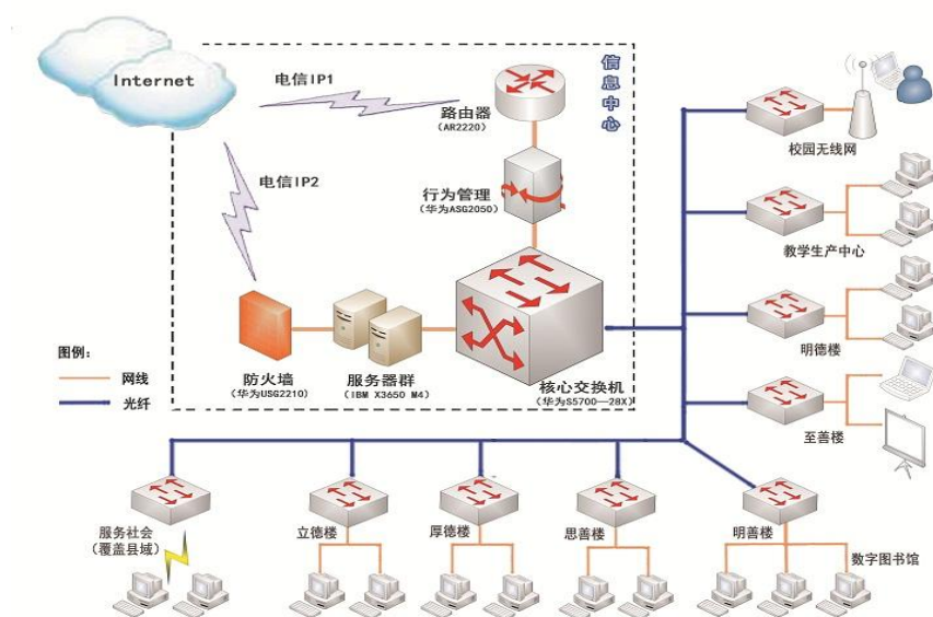
信息化校园网络拓扑结构图
